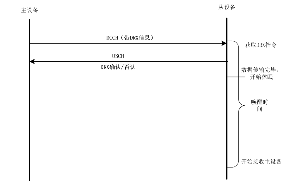
图 11 DRX 过程
