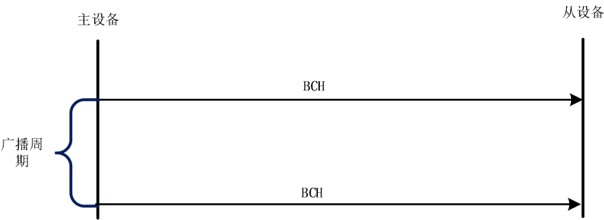
图 7 节点广播过程
