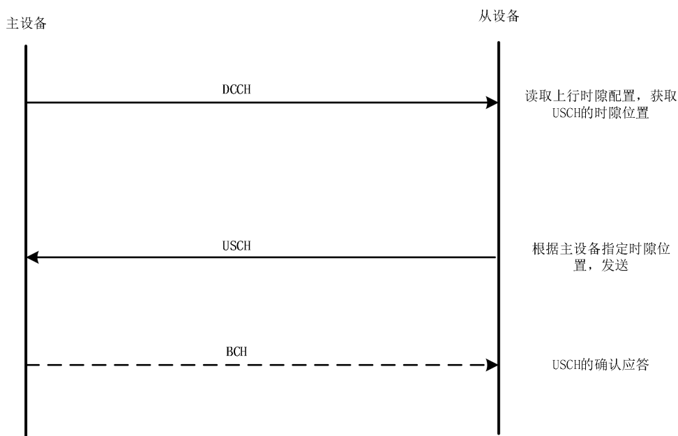
图 10 USCH 的通信过程
