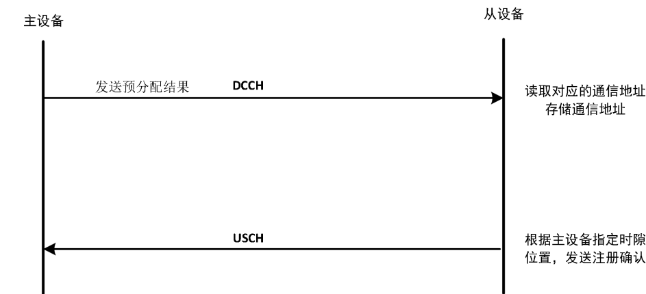
图 9 预分配注册过程
